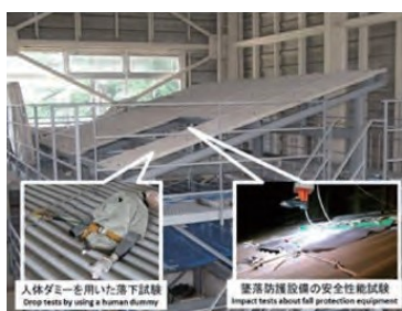
屋根墜落試験装置
